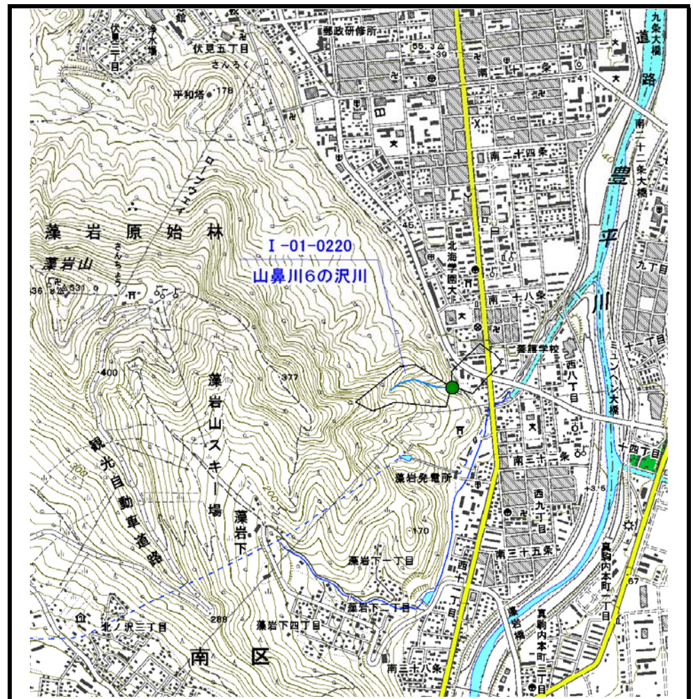
位置図(1/25,000)
