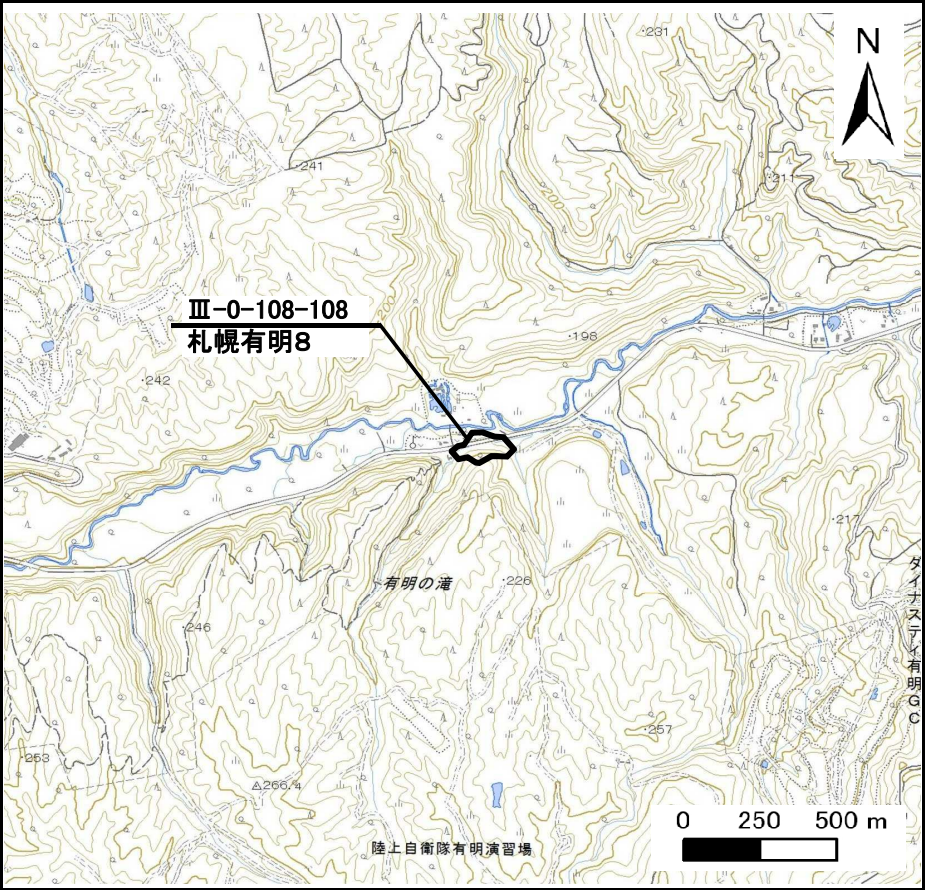
位置図(S=1:25,000)
